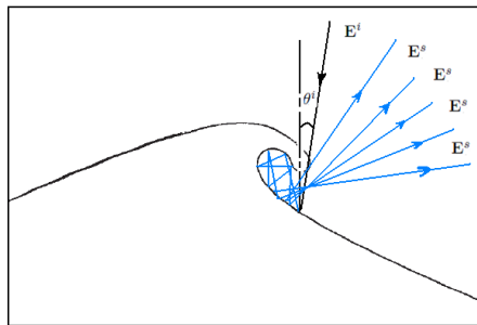
Figure7:Diffusion multi- trajet
