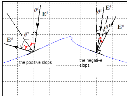
Figure 6 : trajets de la diffusion simple
