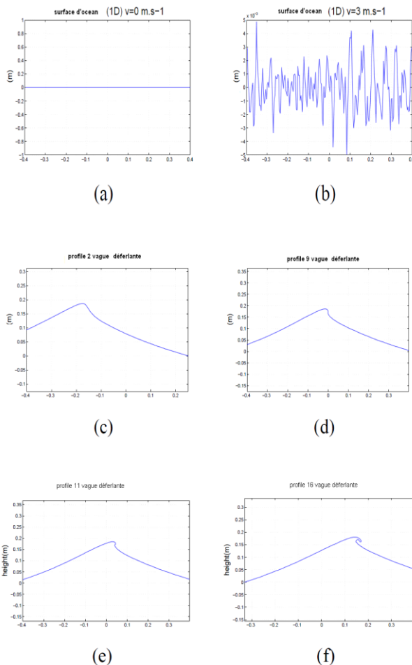
Figure 4 : Différentes phases de construction d'une vague déferlante
