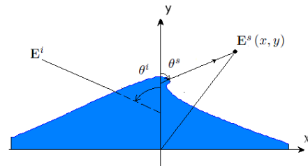
Figure 3: La géométrie de diffusion par une vague déferlante.
