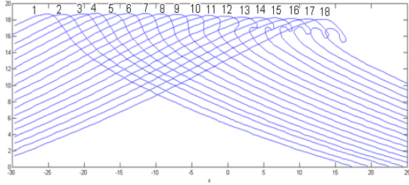
Figure 2 : profils des vagues déferlantes [5]
