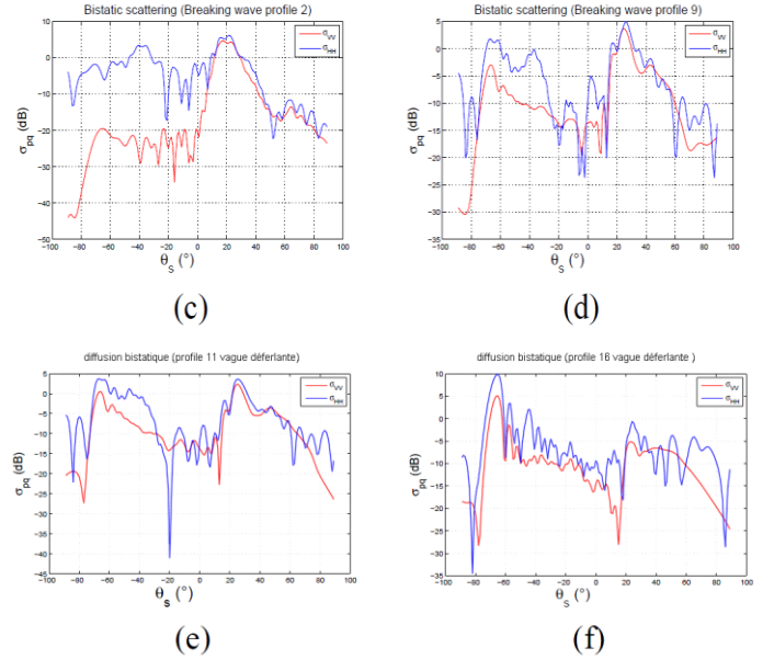
Figure 5 : Coefficients de diffusion bi-statique (polarisation verticale et horizontale \theta_i=-20^\circ )
