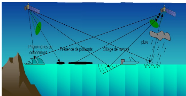
Figure 1 : observation d'une surface maritime hétérogène
